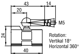
GFK, Magnet Hartferrit Gewicht ca. 30 g Betriebstemperatur: -40 ... +75°C
