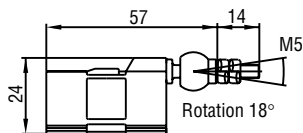
GFK, Magnet Hartferrit Gewicht ca. 30 g Betriebstemperatur: -40 ... +75°C
