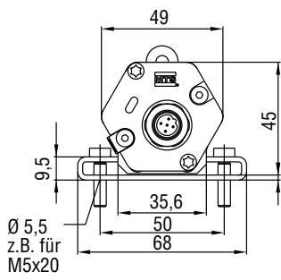
Steckeranschluss D51
