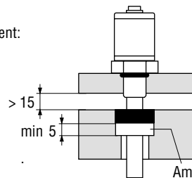
Alternativ: O-Ring 15,3 x 2,2
