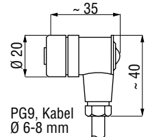
5 pol. 90° Kabeldose M12x1 DeviceNet "Micro", Buchsen Kontakte im 90° Raster drehbar Art. Nr. ST 933 176-100
