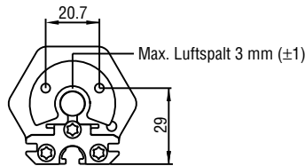
U-Magnet M OD33 Artikel Nr. 251 416-2
