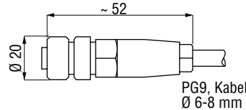
5 pol. Kabeldose M12x1 DeviceNet "Micro", Buchsen Art. Nr. ST 933 171-100
