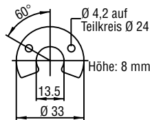
PA-Ferrit-GF20 Gewicht ca. 11g Betriebstemperatur: -40 ... +100°C Flächenpressung max. 90 N/mm 2 Anzugsmoment für M4 Schrauben max. 1Nm
