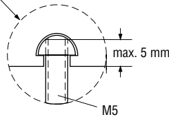
Zapfenmutter in T-Spur
