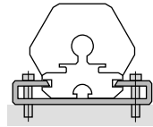
Montageklammer mit Schraube M5 x 20 Anziehmoment: max. 5 Nm
