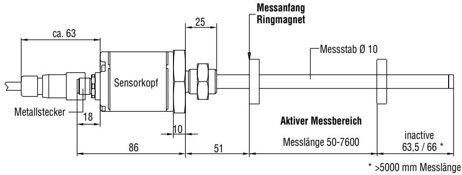
Steckeranschluss D51
